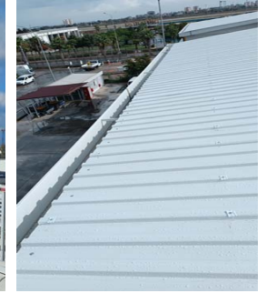
PEGASUS TECHNIC ÇELİK KONSTRÜKSİYON İMALAT VE MONTAJLARI, ÇELİK ÇATI UYGULAMASI, TRAPEZ SAÇ KAPLAMASI ANTALYA HAVALİMANI/ANTALYA
